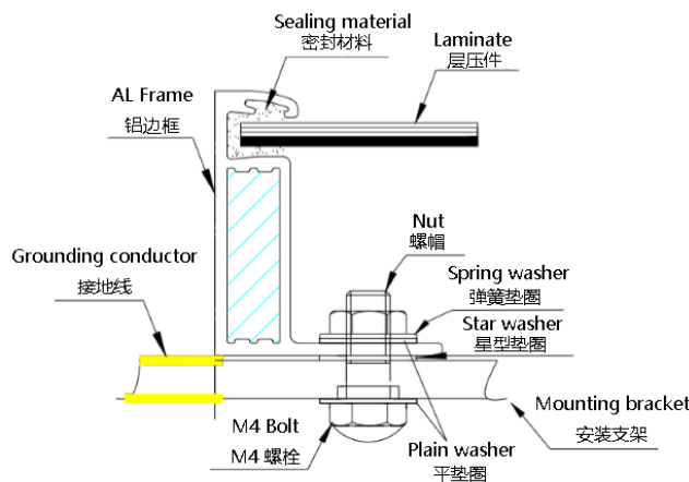
Grounding 接地示意图
